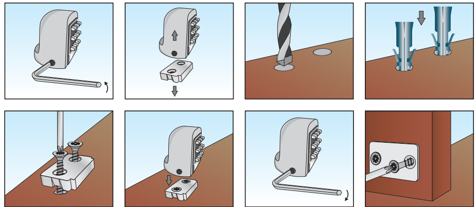
Installation sequece / Instructions de mise en oeuvre / Setzanweisung / Secuencia de instalación / Порядок монтажа
