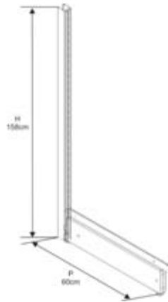
PNT 01 00 158 Uprights for wall stand h 158 cm
